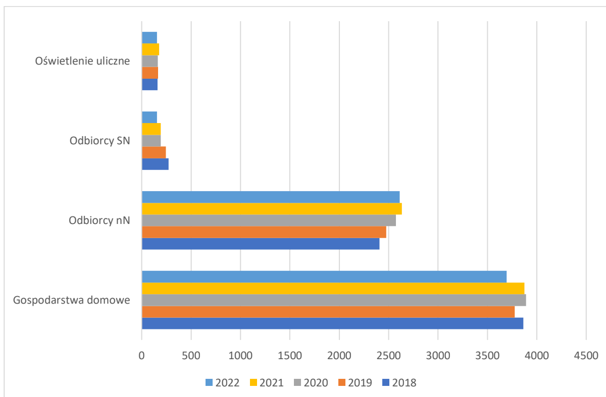
Wykres 6. Zużycie energii elektrycznej [MWh] w podziale na lata dla poszczególnych grup odbiorców w gminie
